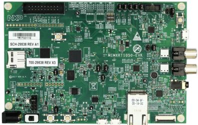
MIMXRT1050 EVK MCU: i.MXRT1050 (Cortex-M7)
