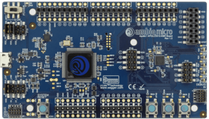
Ambiq Micro Apollo2 EK MCU: Apollo2 (Cortex-M4)
